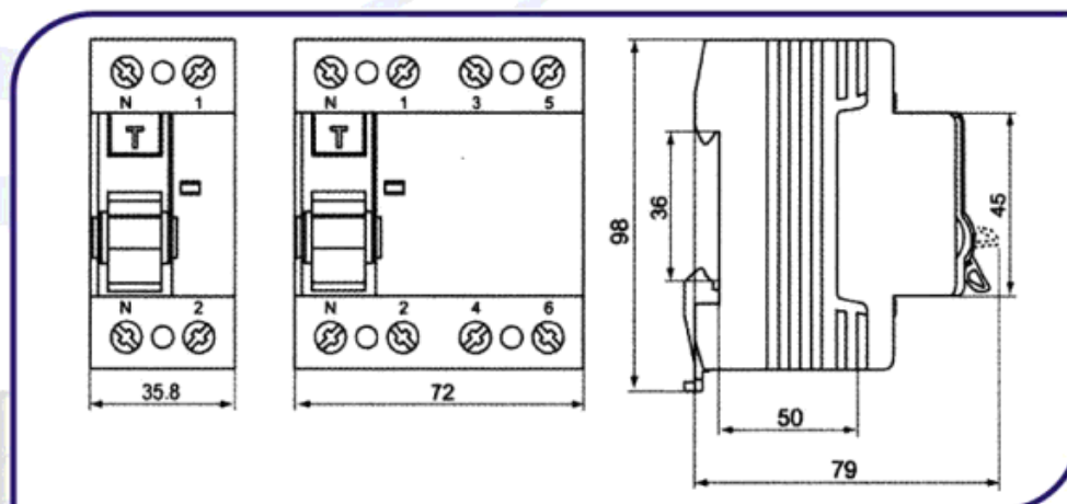
• ابعاد و اندازه کلید محافظ جان مدل PFR
