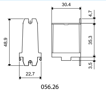
Top 35 mm rail (EN 60715) adaptor for 56.32
