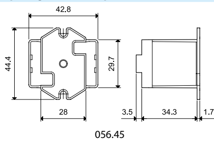
Top 35 mm rail (EN 60715) adaptor for 56.34
