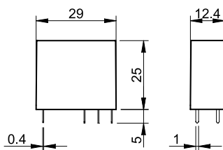
Type 50.12...1000/50.12...5000
